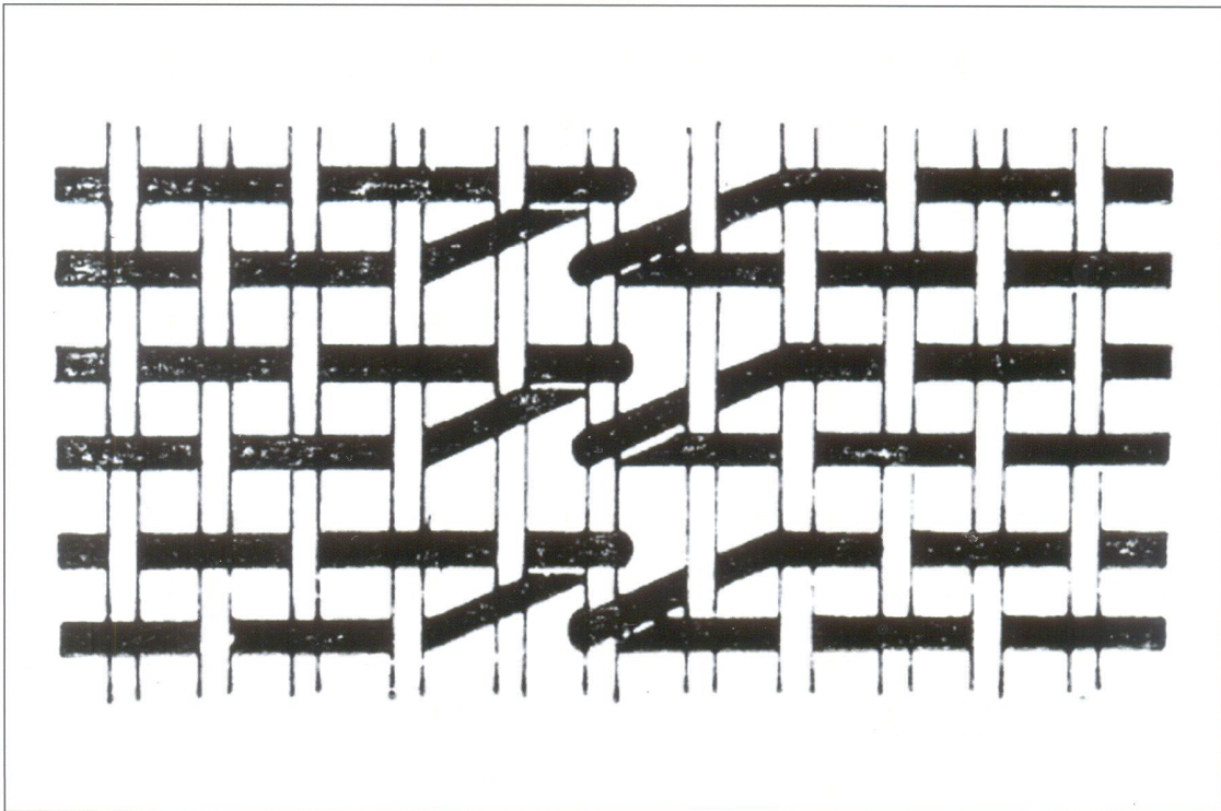
Способы прокидки утка: простое соединение на общую нить основы.
