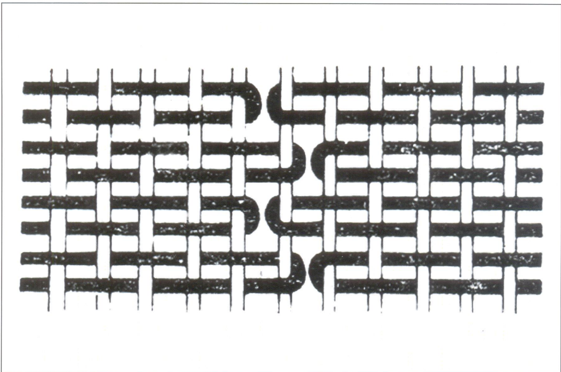
Способы прокидки утка: компенсированное соединение на разные нити основы или паласная техника
