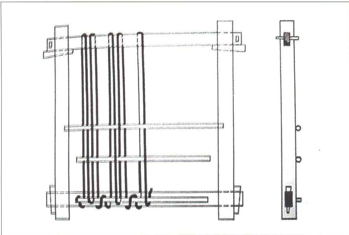
Схема простого вертикального коврикацкого станка.
