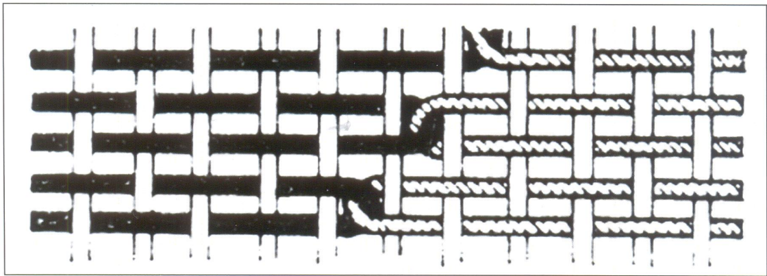
Простое соединение со сцеплением утков между нитями основы.
