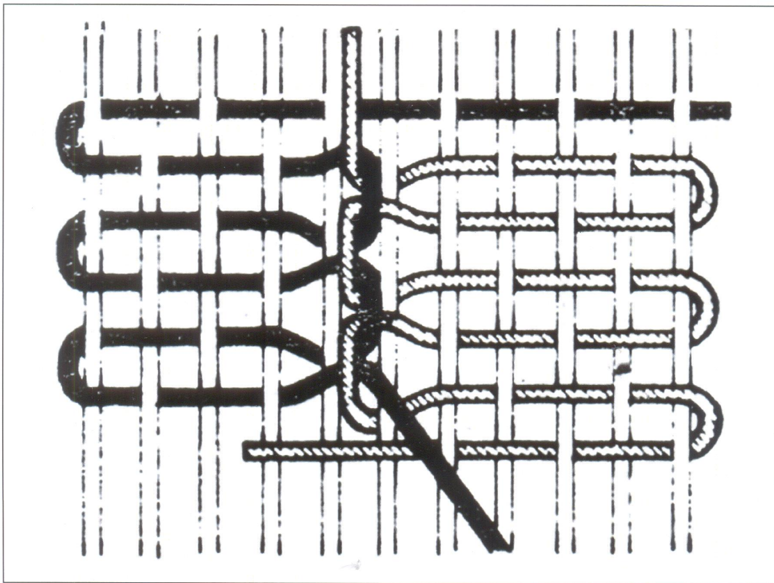
Способы прокидки утка: двойное соединение со сцеплением утков между нитями основы.
