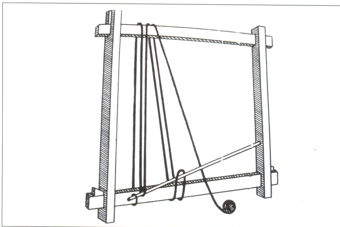
Схема заправки вертикального станка основой.
