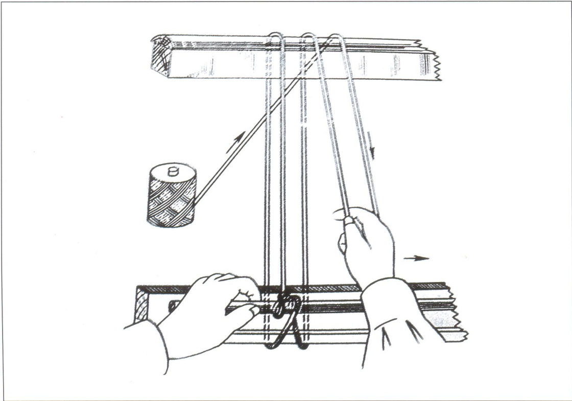
Способ заправки станка основой.
