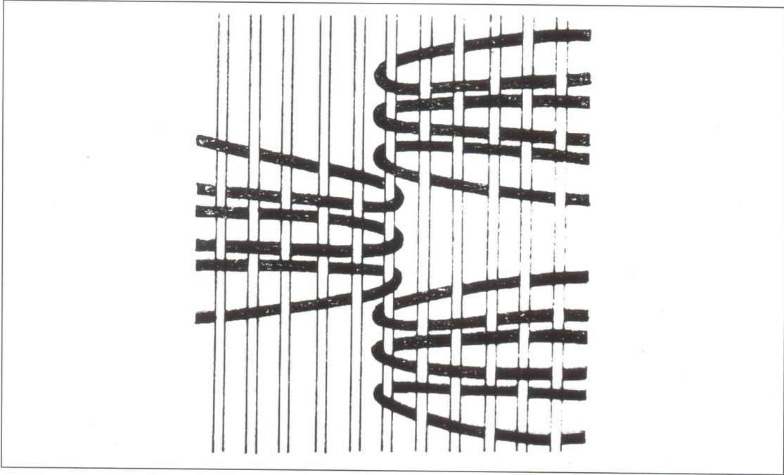
Способы прокидки утка: простое группированное соединение.
